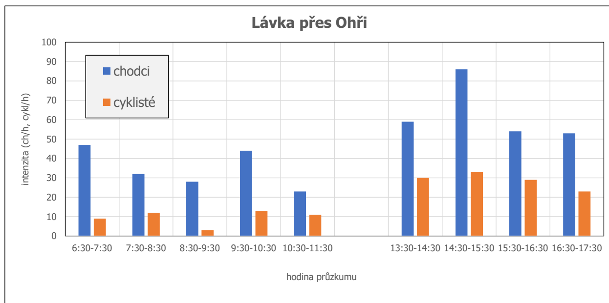
Obrázek: Hodinové intenzity pěších a cyklistů
