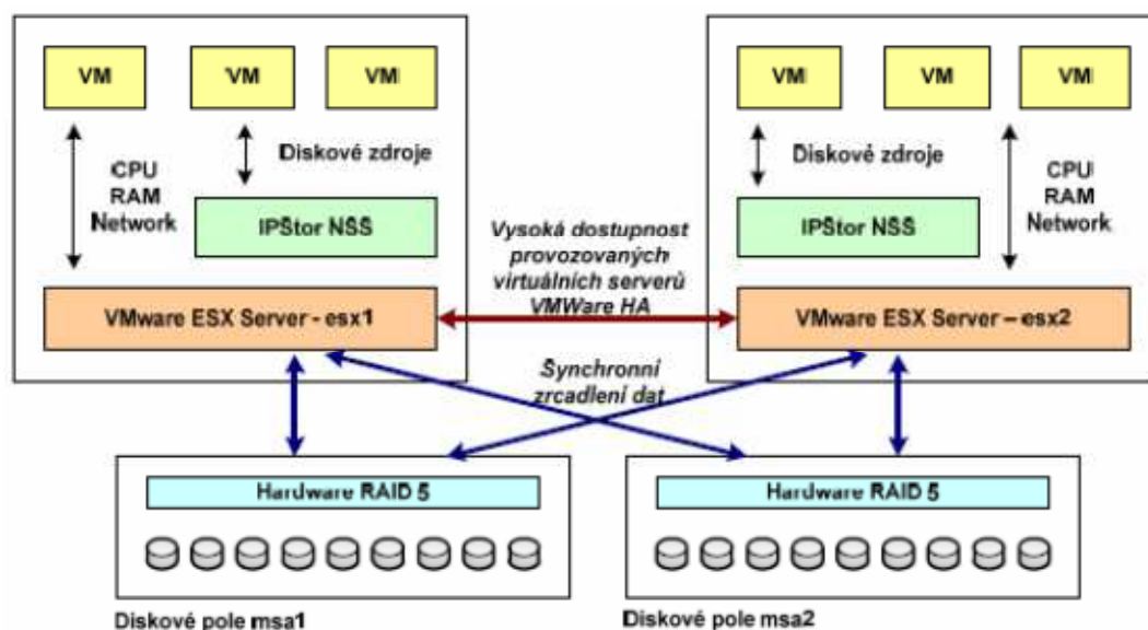
Obrázek 5 – logické schéma diskového subsystému
